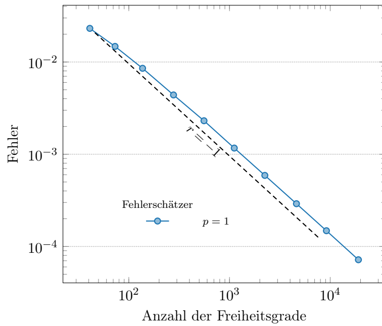
Abbildung 2.3: Numerische Resultate zur singulären Lösung auf dem L-Shape aus Abschnitt 3.1. Wir visualisieren den Fehlerschätzer \eta_\ell über der Anzahl \mathbf{ndof} der Freiheitsgrade.
